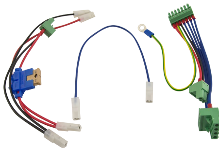
Zestaw wtyków i przewodów
