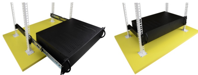
Montaż z szynami ARAS450 do 30kg
