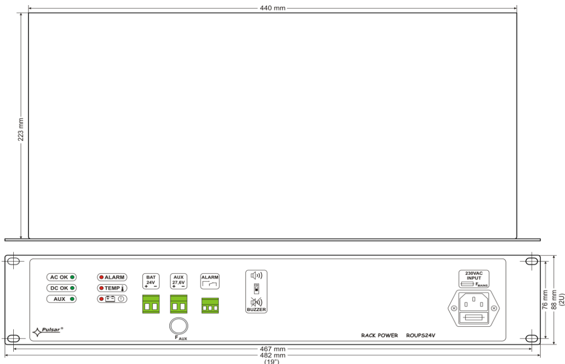
Rys.3. Widok zasilacza.
