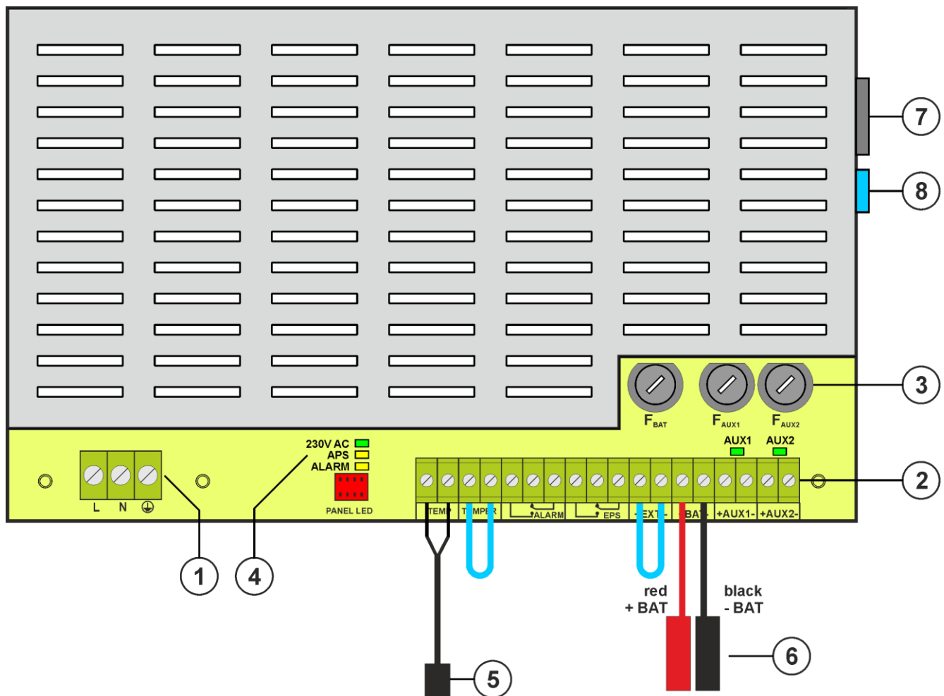
Rys. 2. Widok modułu zasilacza na podstawie EN54C-2A7LCD.
