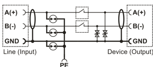
Uproszczony schemat ochronnika
