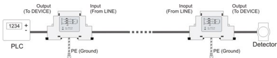
Schemat prawidłowego zabezpieczenia obwodu wejścia / wyjścia
