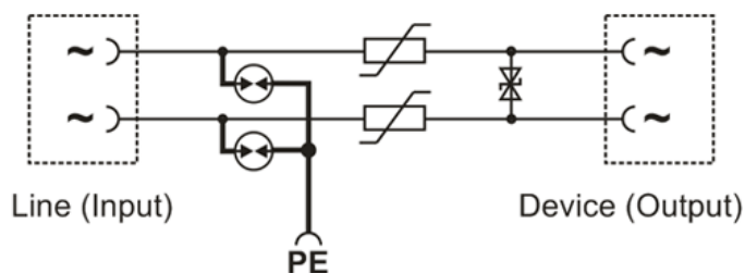
Uproszczony schemat ochronnika
