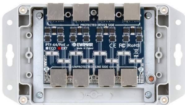
Przykład montażu modułu w obudowie
