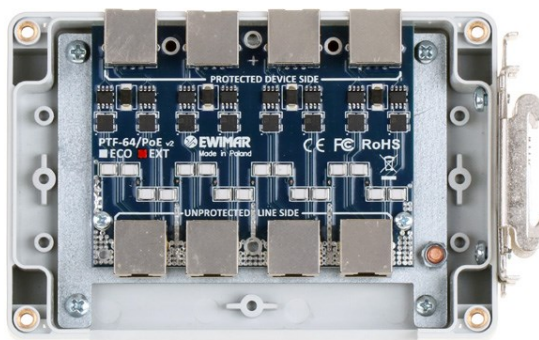
Przykład montażu modułu w obudowie
