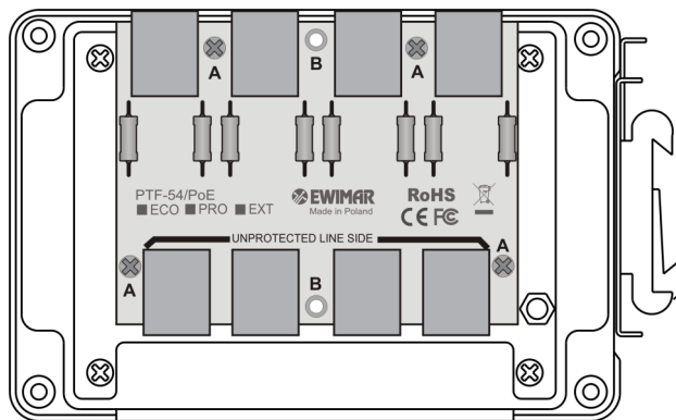
Przykład montażu modułu w obudowie
