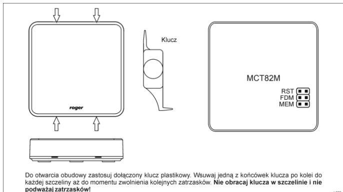
Rys. 3 Sposób otwarcia obudowy czytnika do montażu natynkowego i lokalizacja styków serwisowych
