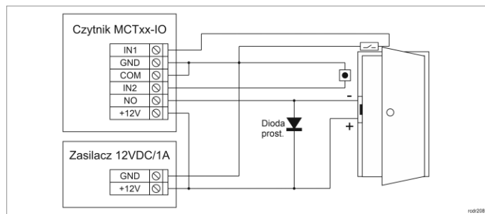
Rys. 6 Podłączenie zamka, czujnika otwarcia drzwi i przycisku wyjścia do czytnika MCT82M-IO-HR
