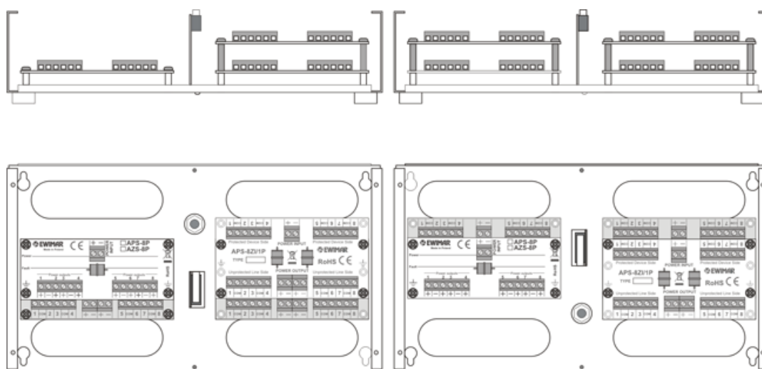
Przykład montażu modułów ochronnych APS i AZS
